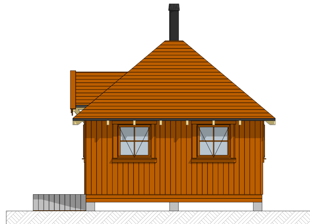
1:50 Fasade Øst
