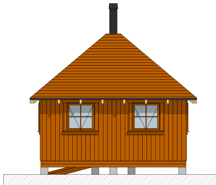
1:50 Fasade Nord
