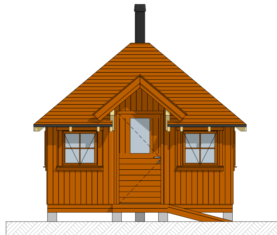
1:50 Fasade Sør
